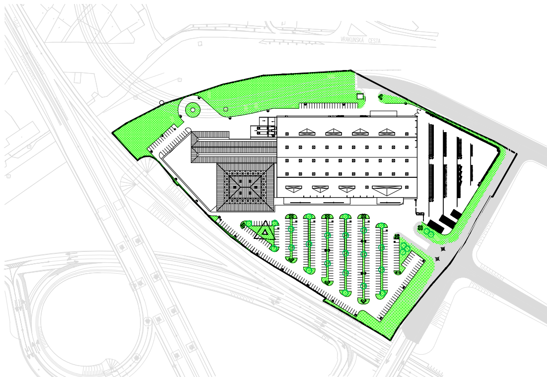
GRUNDRISS
