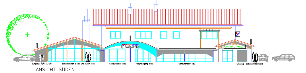
ANSICHT SÜDEN
