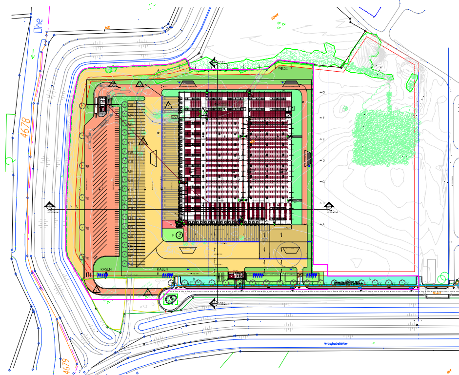
LAGEPLAN
