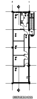
OBERGESCHOSS
