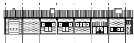
ANSICHT VON OSTEN
