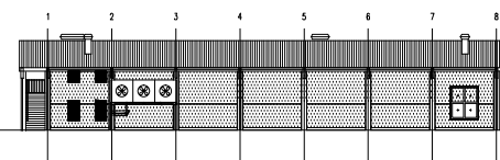
ANSICHT VON WESTEN
